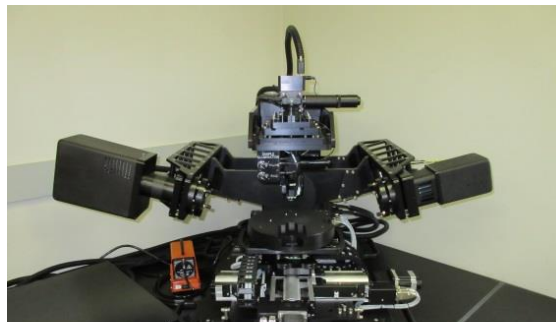
分光エリプソメーター M-2000UI
